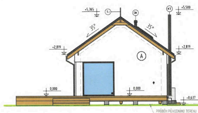
POHLED ZÁPAD:
