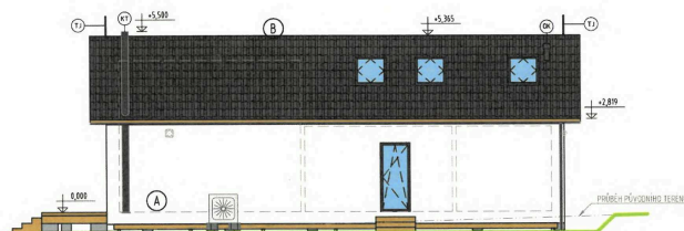
POHLED SEVER:
