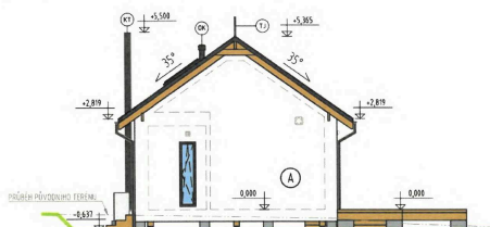
POHLED ZÁPAD:
